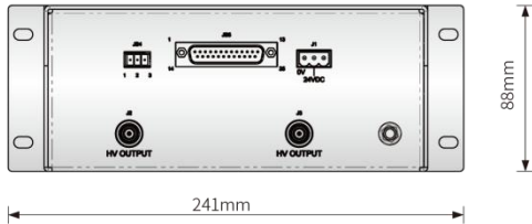
后视图
