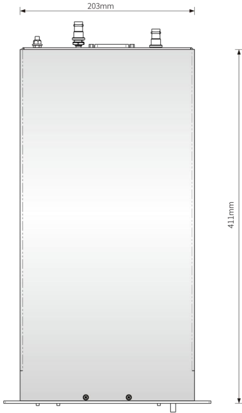
俯视图
